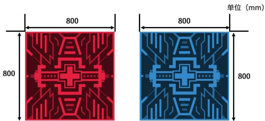
图 3.3-2 启动区俯视尺寸图
