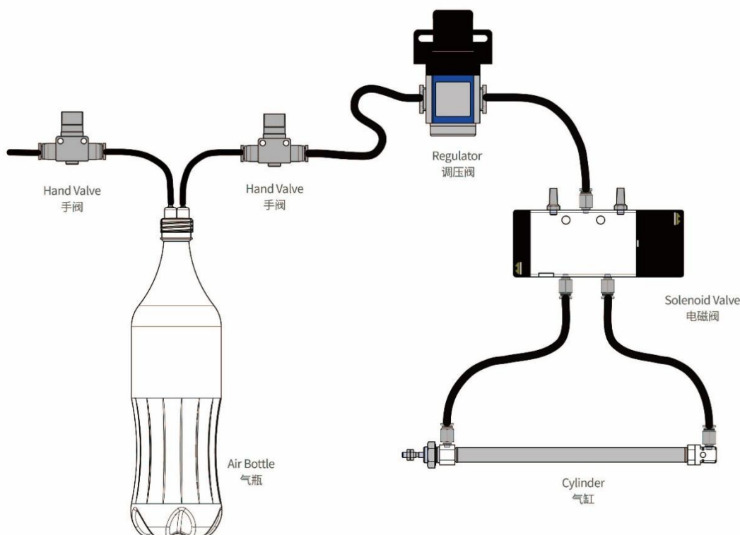
图 4.3-1 单缸气动装置的标准连线图
