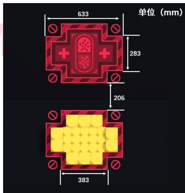
图 3.3-7 药剂摆放区尺寸图
