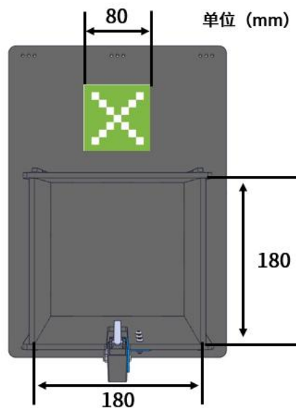
图 3.4-6 方形槽示意图
