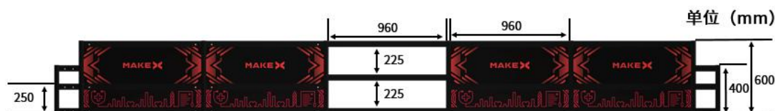
图 3.3-5 中央隔栏尺寸图
