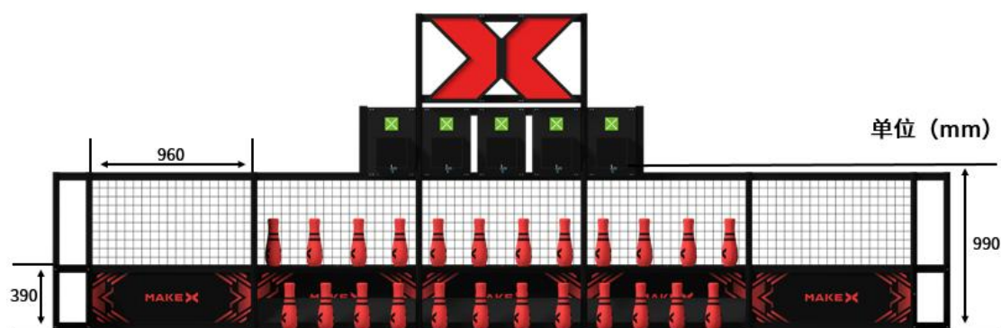
图 3.3-4 病毒隔离区前视尺寸图
