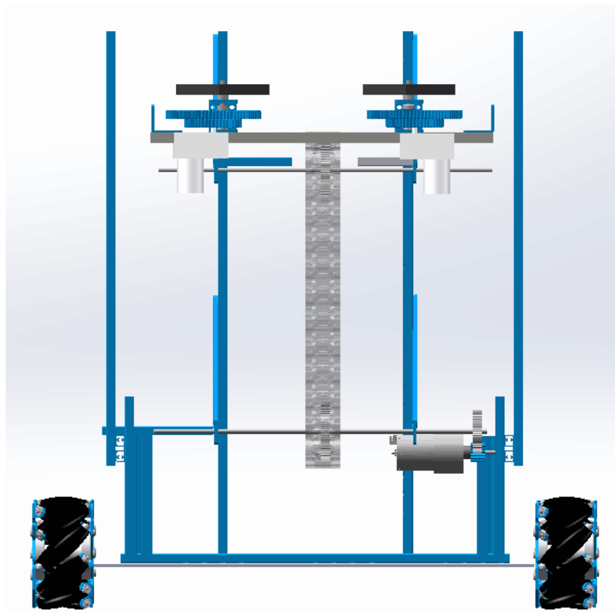
机械正视图
