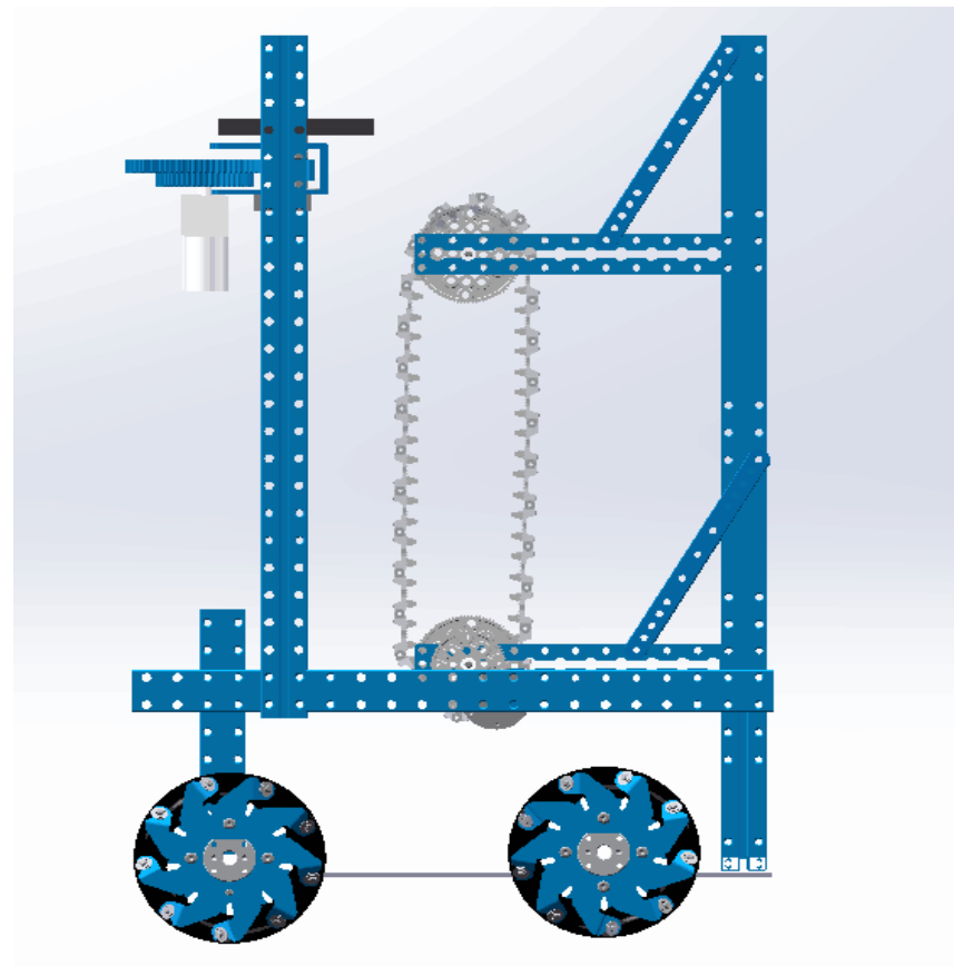
机械侧视图
