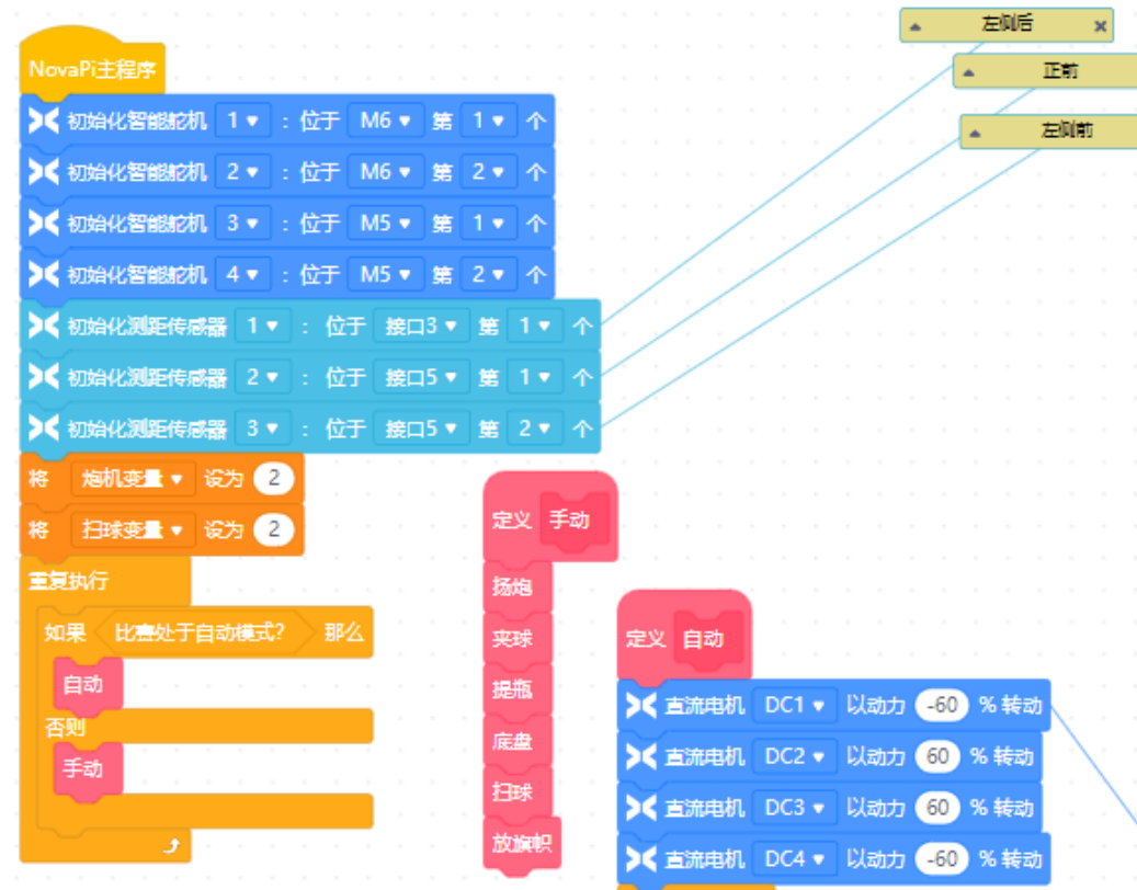
总程序架构
